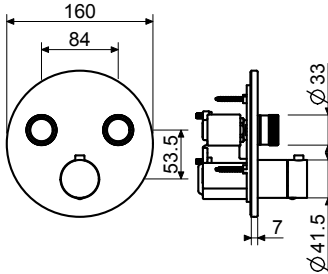
PRO003EDEN Prolunga vedi pag. 328 Extension see page. 328
