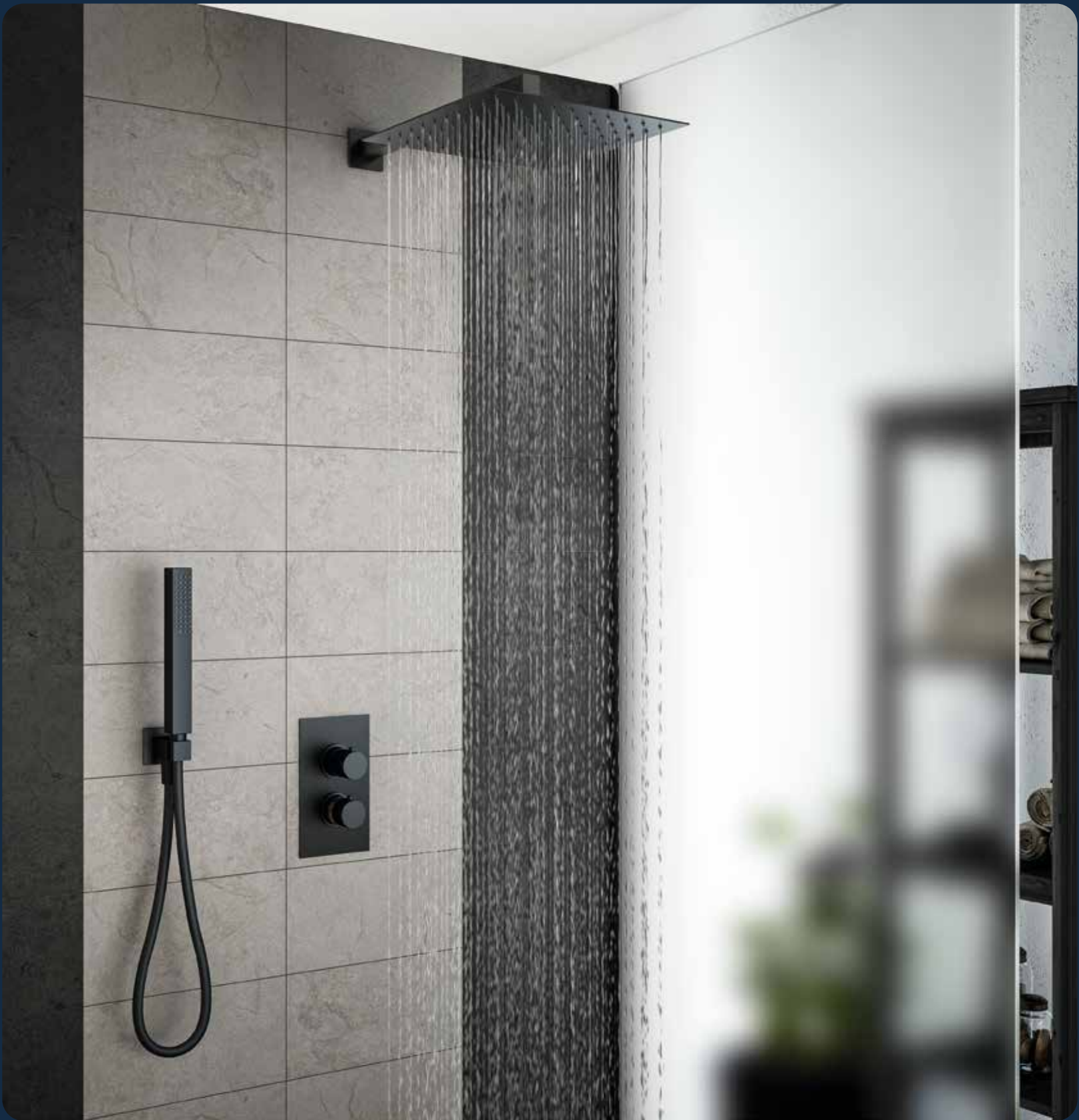
WLSKIT8-CR — Soffione in acciaio 250x250 mm con valvola di sicurezza. Braccio doccia L 300mm. Set doccia con presa acqua duplex, doccetta in ABS e flessibile. Finitura Nero Opaco
