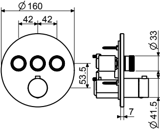
PRO003EDEN Prolunga vedi pag. 328 Extension see page. 328
