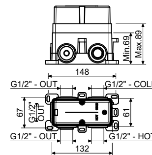
Scatola incasso Handy Box per miscelatore Ø35 con deviatore 2-3 uscite Single-lever mixer for concealed installation with 2-3-outlet diverter, Ø 35 mm
