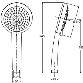
Doccia idromassaggio anticalcare 3 getti in ABS con sistema risparmio acqua fino al 30%. 3-jet hydromassage hand shower in ABS with antiscale, saves up to 30% waste water.
