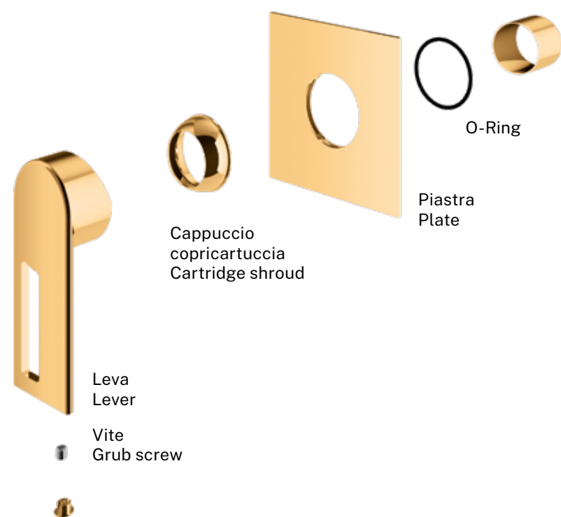
Copertura cartuccia Cartridge cover cap
