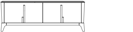
Art. CMP/5 Base 2 cestoni maniglie legno L. 150 P. 56 H. 54,3
