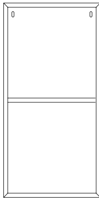
Art. MEL57 Pensile verticale 2 vani L.59 P.36 H.118
