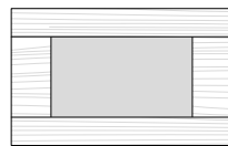
Art. MEL44 Telaio vetro orrizontale apertura vasistas L.58,6 H.36,6 Sp.2,5
