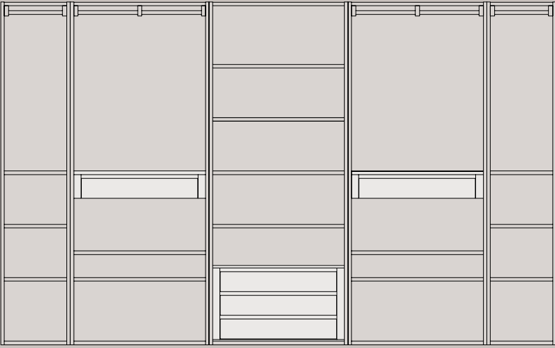
Art. M6130 Proposta cabina armadio vista aperta. L. 400 P. 59 H.247
