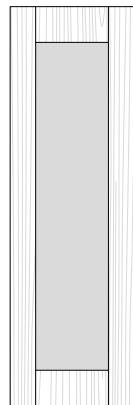
Art. MEL29 Telaio vetro verticale. L.36,6 H.117,6 Sp.2,5
