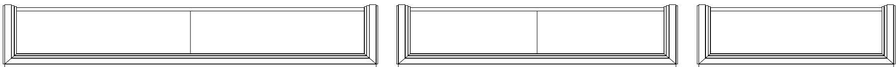
Art. MEL1 Base 2 cestoni. L.224 P.53 H.38
