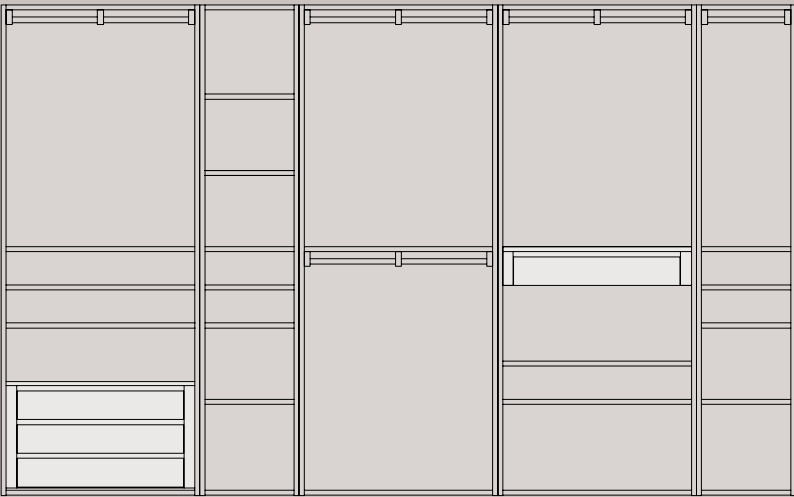
Art. M6128 Proposta cabina armadio vista aperta. L. 400 P. 59 H.247
