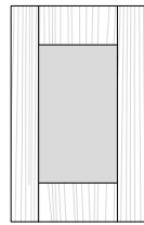
Art. MEL33 Telaio vetro verticale. L.36,6 H.58,6 Sp.2,5
