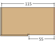
Angolo/Corner Art. Y120 con porte. Art. Y120/S senza porte. Armadio angolo 90°
