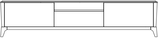
Art. CMP/3 Base 3 cestoni 1 vano. L. 236 P. 56 H. 54,3
