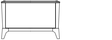
Art. CMP/11 Base 1 cestone. L. 83,5 P. 56 H. 54,3
