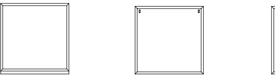
Art. CMP/28SX - Art. CM- P/29DX Base per anta. L.59 P. 58 H. 61,5
