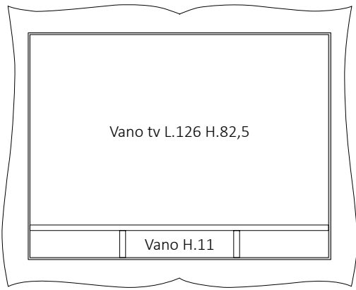
Art. MCM5 Modulo porta tv con cornice L.148 P.34 H.118
