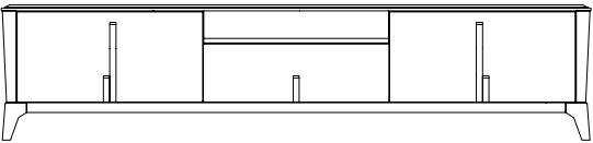
Art. CMP/2 Base 3 cestoni 1 vano maniglie legno. L. 236 P. 56 H. 54,3
