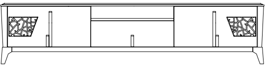
Art. CMP/1 Base 3 cestoni 1 vano maniglie legno e traforo. L.236 P. 56 H. 54,3
