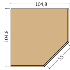
Angolo/Corner Art. Y122 con porte. Art. Y122/S senza porte. Armadio angolo 45°
