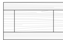
Art. MEL35 Telaio legno orrizontale apertura vasistas L.58,6 H.36,6 Sp.2,5
