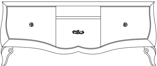
Art. MCM3 Base 3 cassetti 1 vano liscia L.155 P.55 H.63
