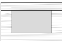
Art. MCM36 Anta a telaio vetro orizzontale ap. vasistas L.58,6 H.36,6 Sp.2,5
