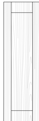
Art. MEL28 Telaio legno verticale. L.36,6 H.117,6 Sp.2,5
