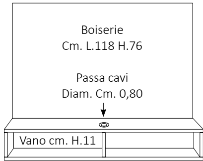
Art. MEL9 Boiserie con porta tv e video L.118 P.35 H.91
