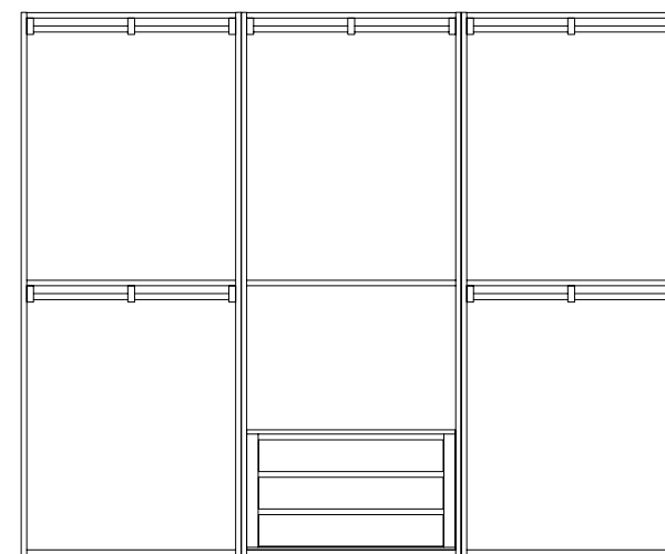
Armadio/Wardrobe Art. M6061 Frassino 6 ante battenti con maniglie legno. L. 300 P. 61,5 H. 247
