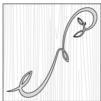
Art. MEL45sx Decoro verticale L.58,6 H.58,6 Sp.2,5
