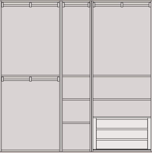
Art. M6133 Proposta cabina armadio vista aperta. L. 250 P. 59 H.247
