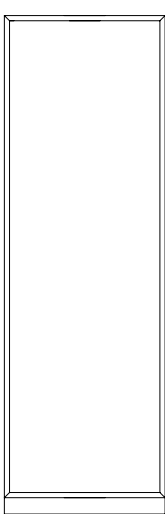
Art. MCP30 Colonna 1 vano. L.59 P.36 H.183
