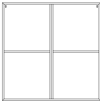
Art. MCP44 Pensile cubo 4 vani. L.118 P.36 H.118
