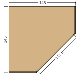
Angolo/Corner Art. Y123 con porte. Art. Y123/S senza porte. Armadio angolo 45°
