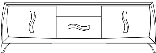
Art. MCP17 Base 3 cestoni lisci e vano. L.189 P.57 H.60
