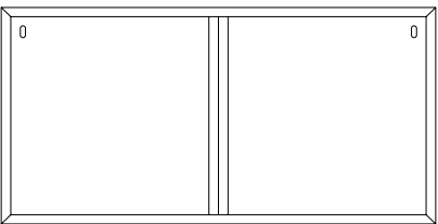
Art. MCM6 Pensile orizzontale 2 vani L.118 P.36 H.59
