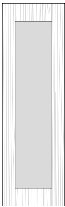
Art. MCM39 Anta a telaio vetro verticale L.36,6 H.117,6 Sp.2,5
