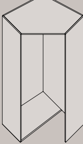
Art. MCB 3/SX - Art. MCB4/DX Struttura angolo con spogliatoio passo ripiani in H.16,7 cm. cm. 132/132 X 133/59 H.247
