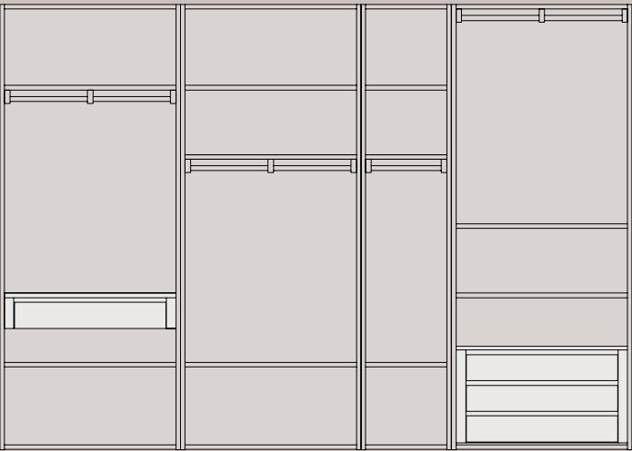
Art. M6131 Proposta cabina armadio vista aperta. L. 350 P.X 59 H.247
