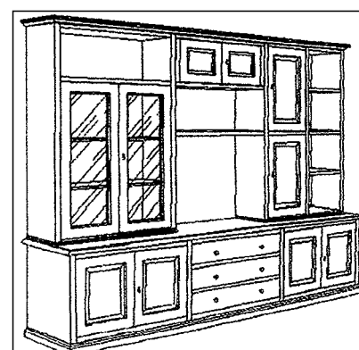
Art. E6012 Parete Volterne Living room Стеллаж L 296 P 50 H 226 - m³ 2,50
